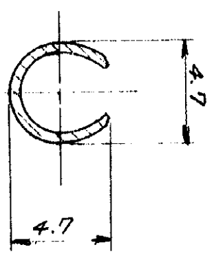
断面 B-B
